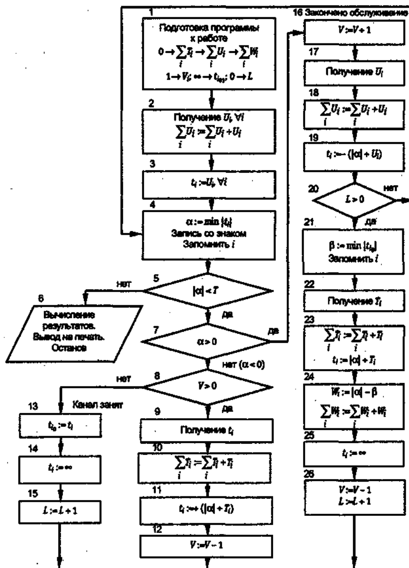
Рис. 13.12. Моделирующий алгоритм: T_i — глубина моделирования; L — длина очереди на обслуживание
